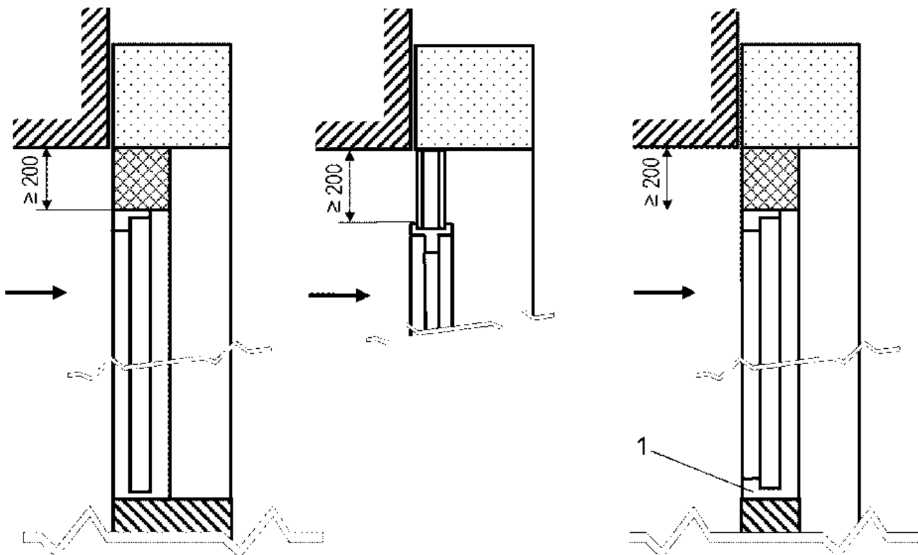
Рисунок 6. Схемы монтажа образцов распашных дверей(вертикальное сечение)
