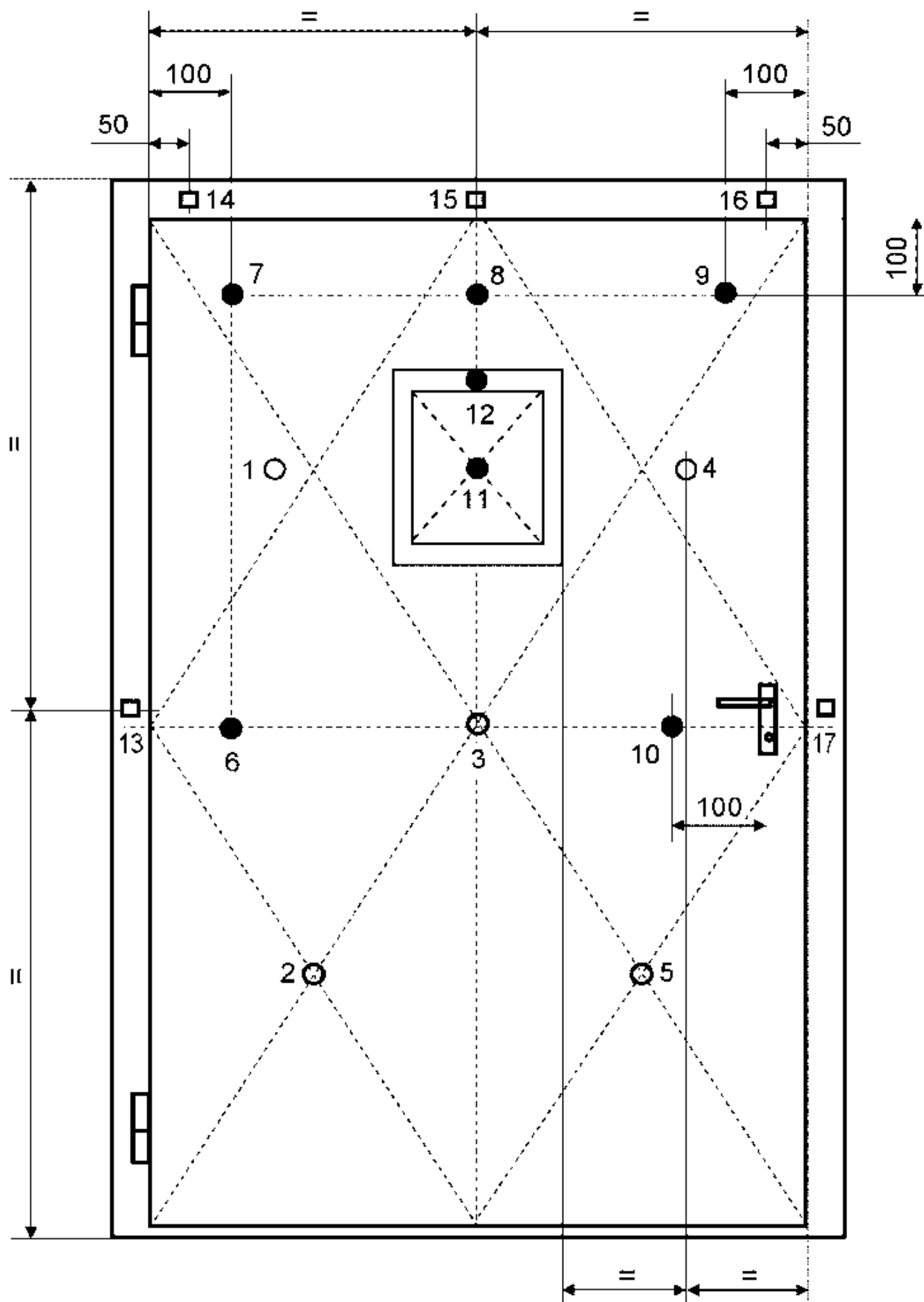
Рисунок 22. Схема установки термодатчиков на необогреваемой поверхности распашных двупольных ворот со встроенной дверью
