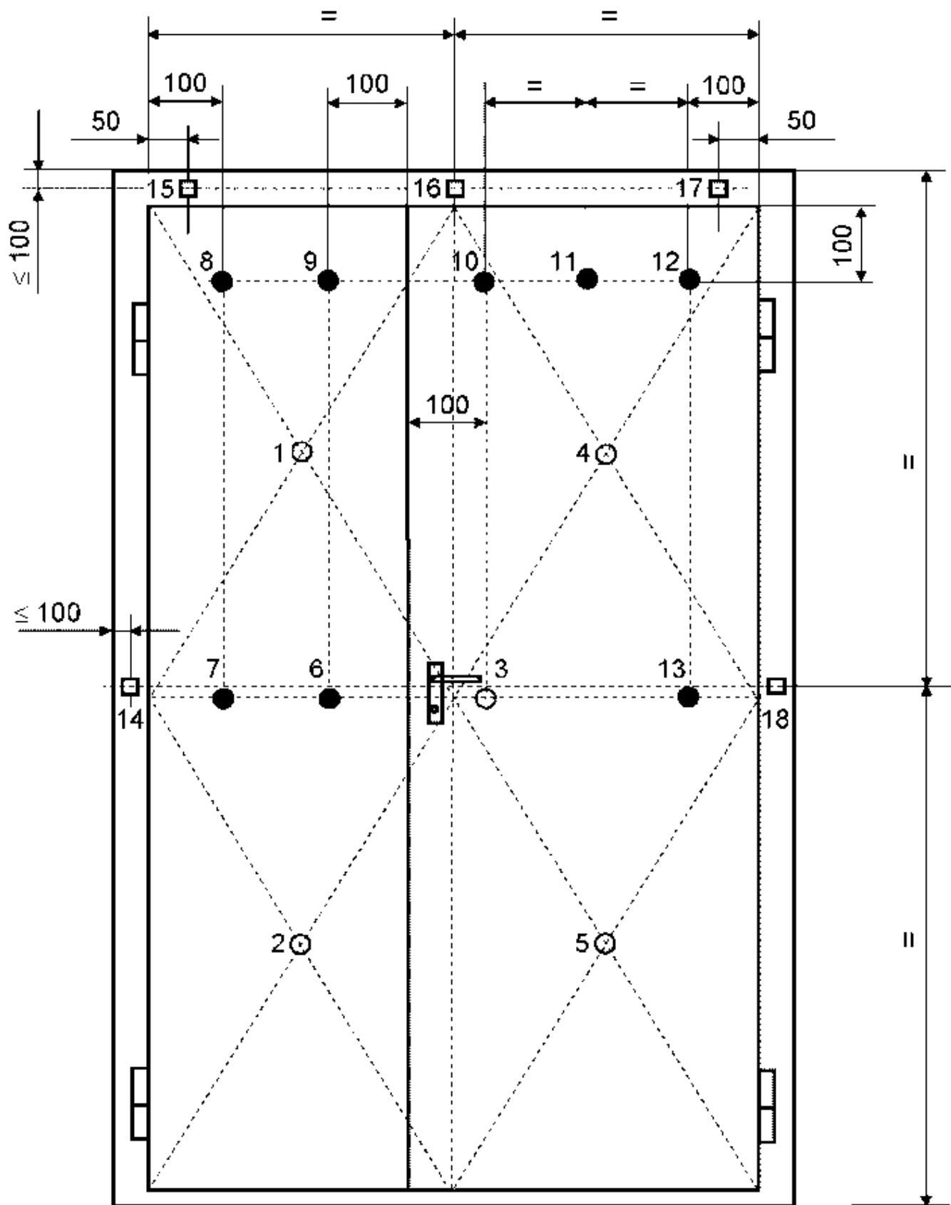
Рисунок 12. Схема установки термодпар на необогреваемой поверхности полотна распашной однопольной двери в зоне 100 мм от его торцевых поверхностей и проема в свету (горизонтальное сечение)
