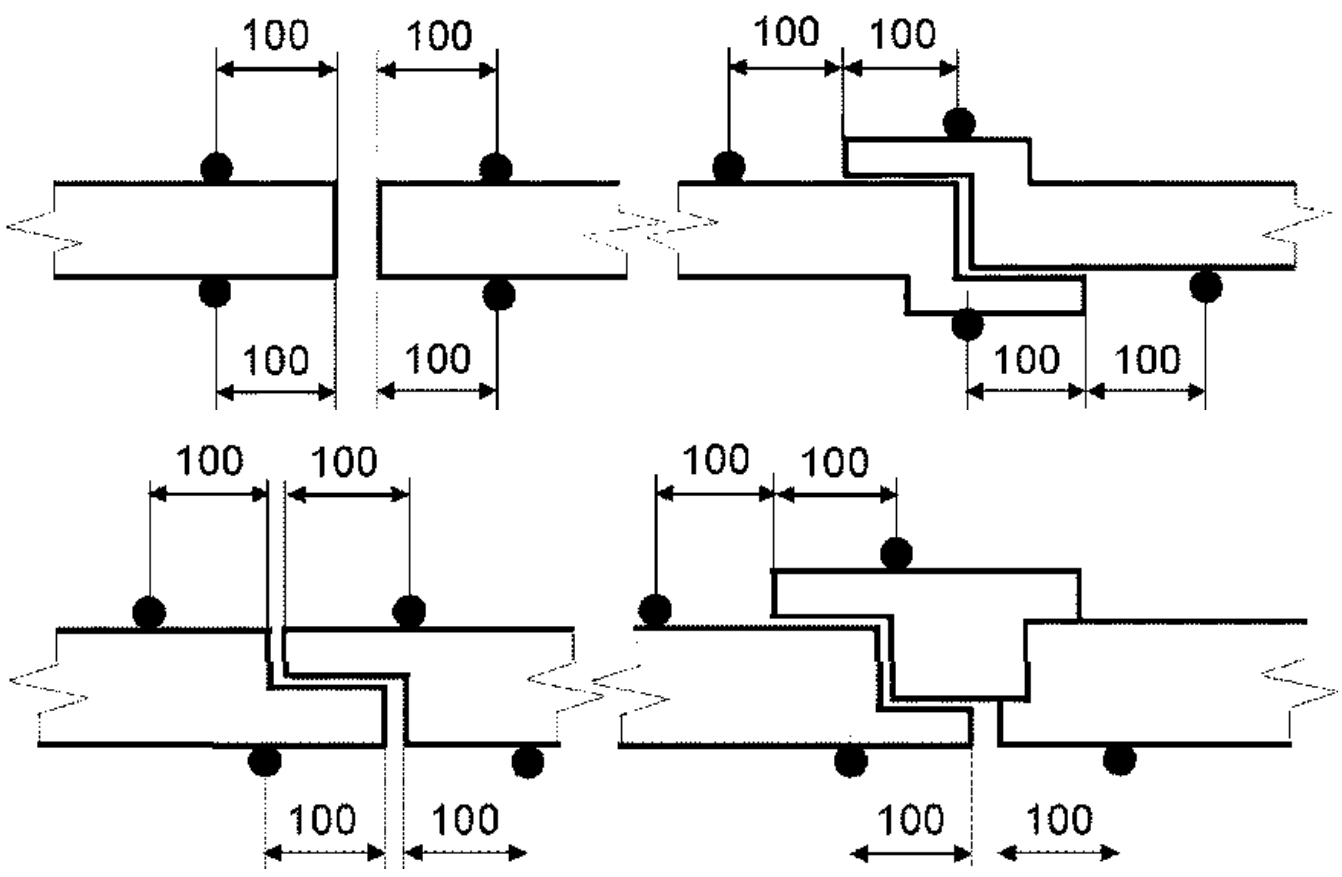
Рисунок 13. Схема установки термодатчиков на необогреваемой поверхности полотен распашной двупольной двери в районе среднего притвора (горизонтальное сечение)
