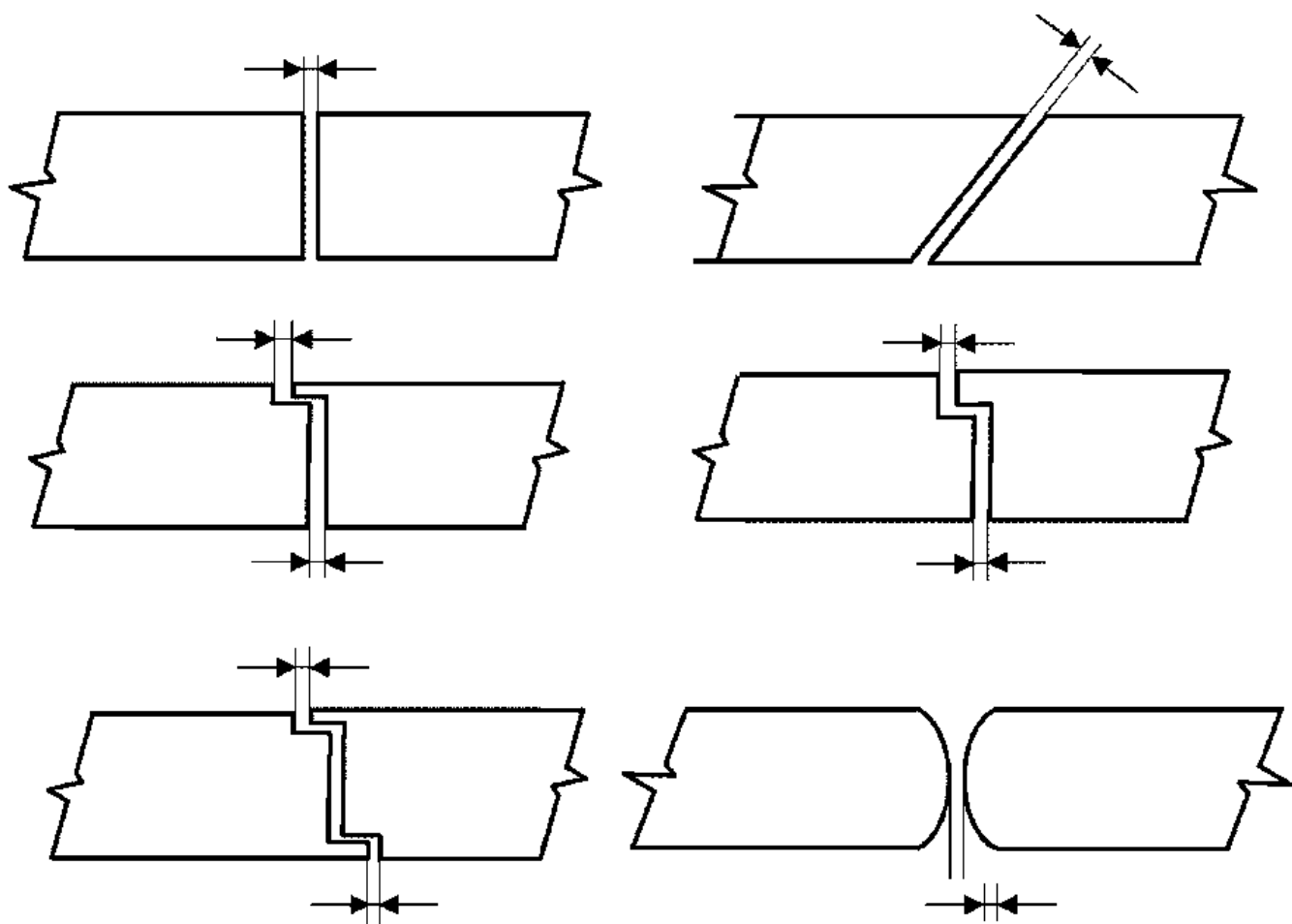
Рисунок 26. Примеры замеров зазоров (горизонтальное сечение)
