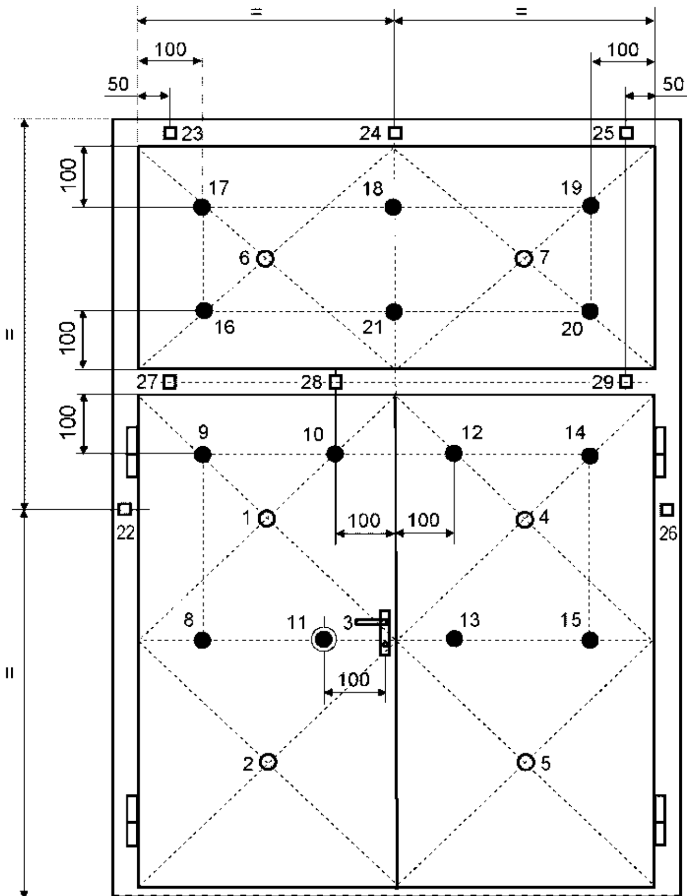
Рисунок 20. Схема установки термодпар на необогреваемой поверхности распашной двупольной двери с фрамугой в зоне 100 мм от торцевых поверхностей коробки (вертикальное сечение)
