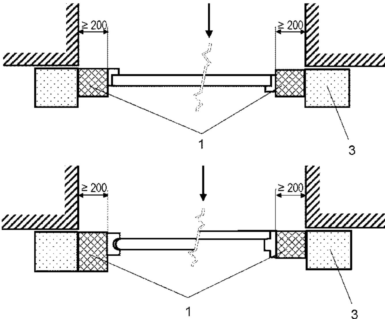
Рисунок 5. Схемы монтажа образцов распашных дверей (горизонтальное сечение)
