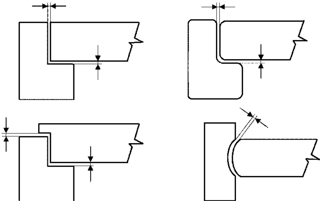
Рисунок 25. Примеры замеров зазоров распашных дверей (горизонтальное сечение)
