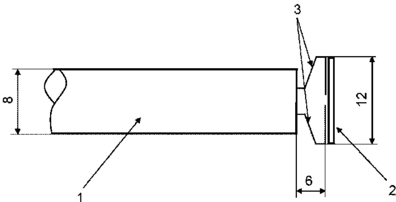
Рисунок 1. Конструкция переносной термопары
