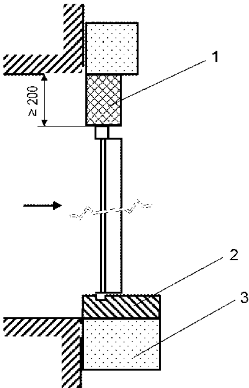
Рисунок 8. Схема монтажа образцов складывающейся двери
