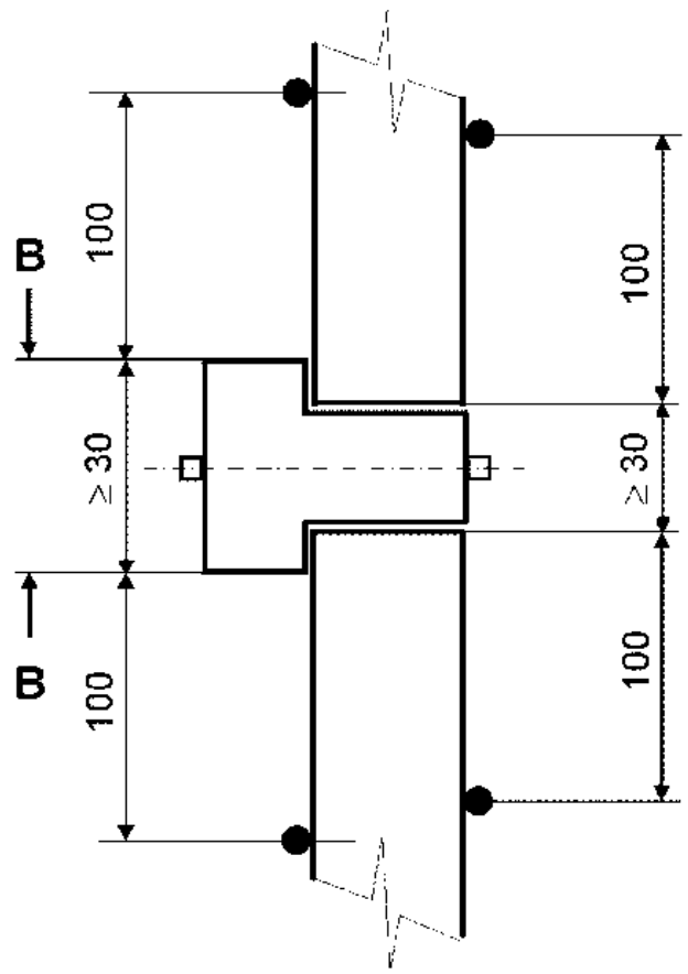
Рисунок 21. Схема установки термодатчиков на неотапливаемой поверхности распашной однопольной двери с частичным остеклением
