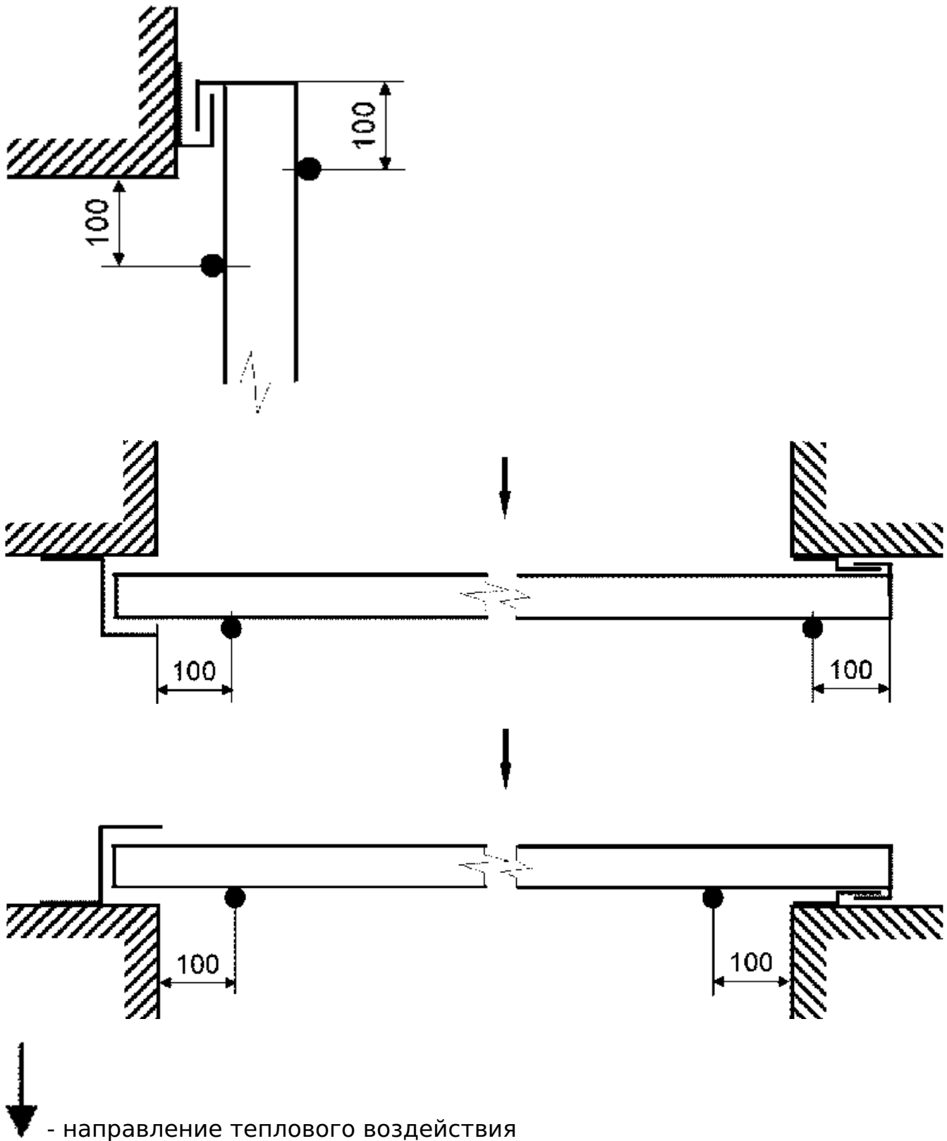
Рисунок 16. Схема установки термодатчиков на необогреваемых поверхностях полотен подъемных и скручивающихся ворот
