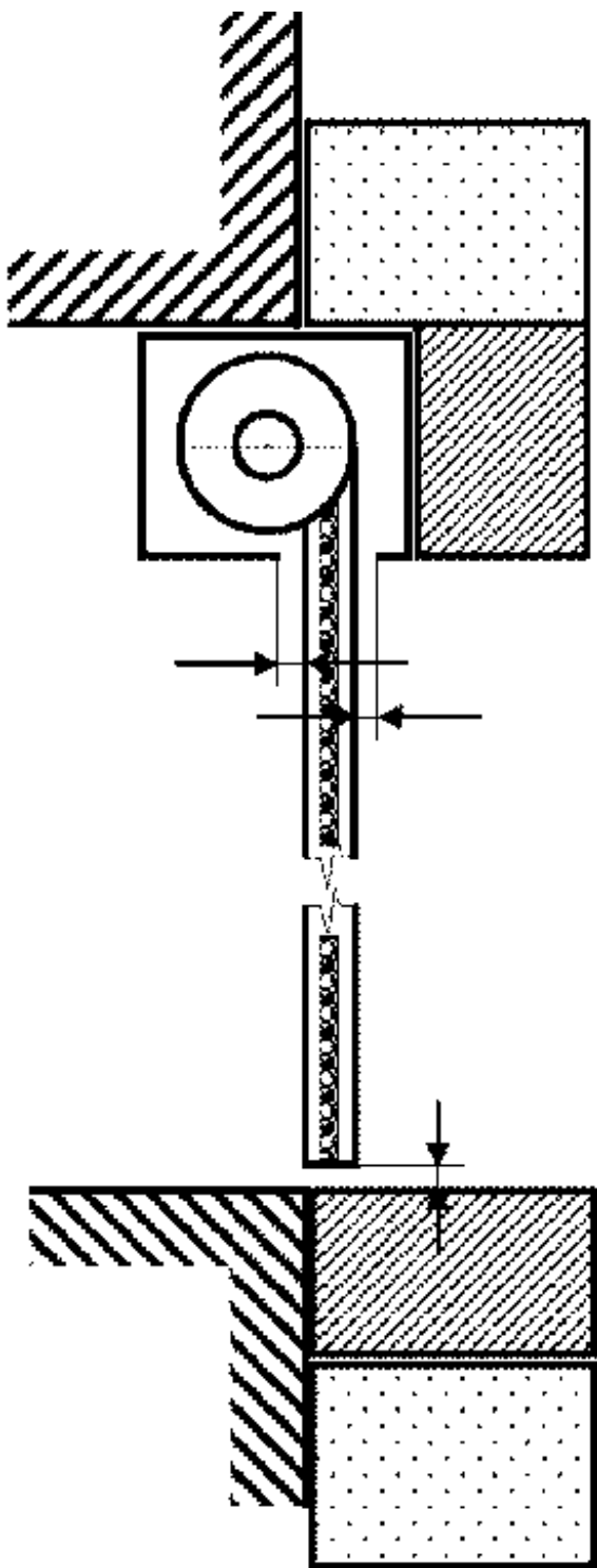
б - подъемные, скручивающиеся ворота
